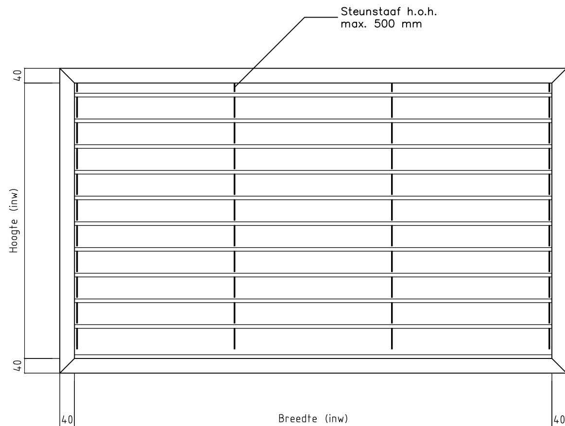
Vooraanzicht
